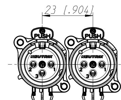
min. Einbauabstand min assembling distance
