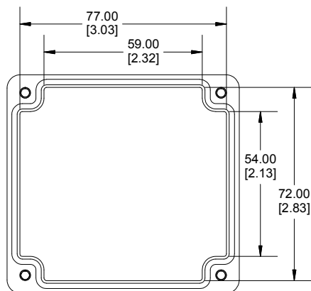
INSIDE LID
