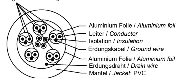
Aderquerschnitt / Wire cross section
