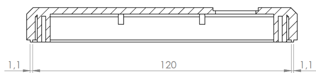
Sección/Section N-N
