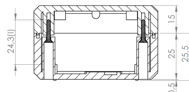
Sección/Section P-P
