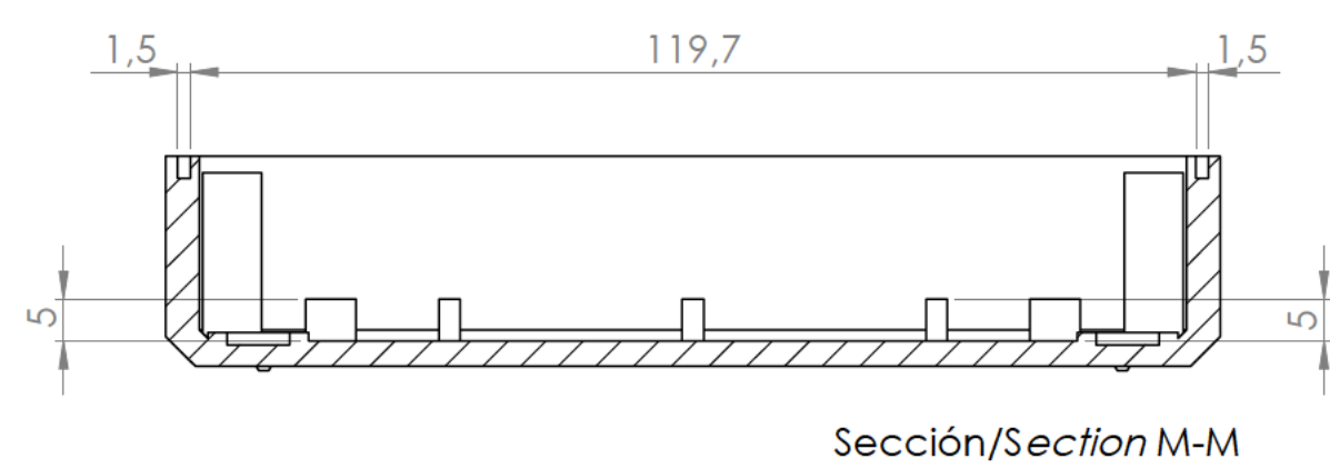
Sección/Section M-M
