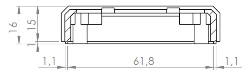
Sección/Section O-O
