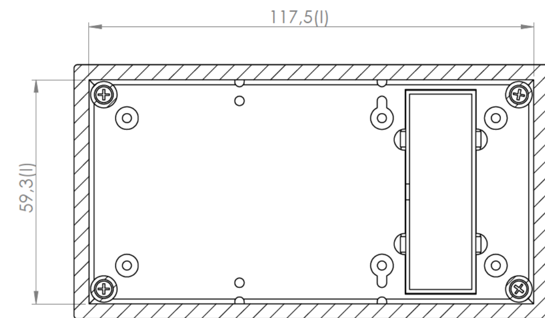
Sección/Section Q-Q
