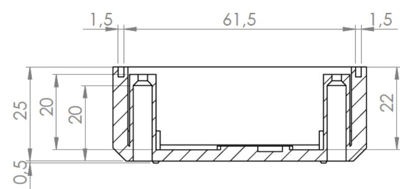
Sección/Section L-L
