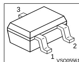
PG-SOT-323
