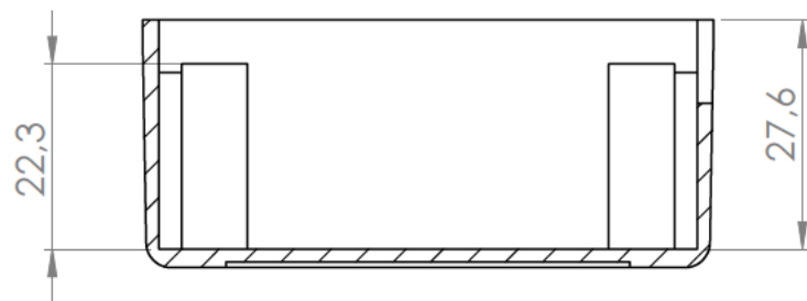
Sección /Section L-L
