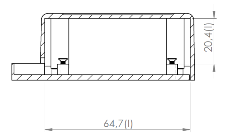
Sección /Section M-M
