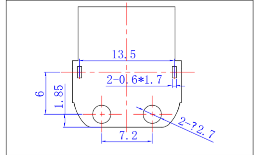
安装尺寸示意图
