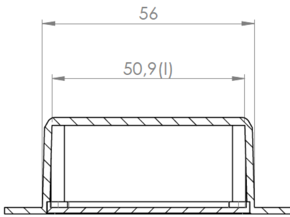
Sección/Section N-N
