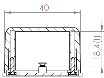
Sección/Section M-M
