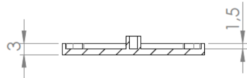
Sección/Section K-K
