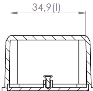
Sección/Section O-O
