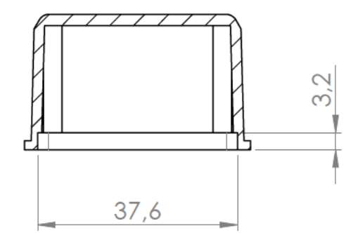
Sección/Section L-L
