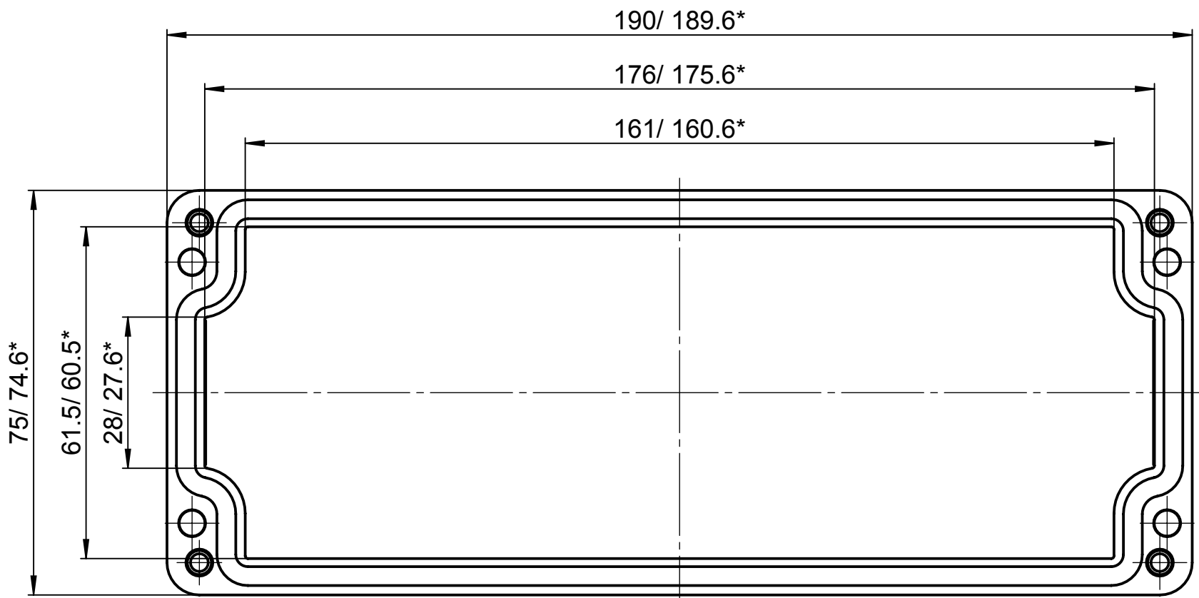
Deckel / Lid
