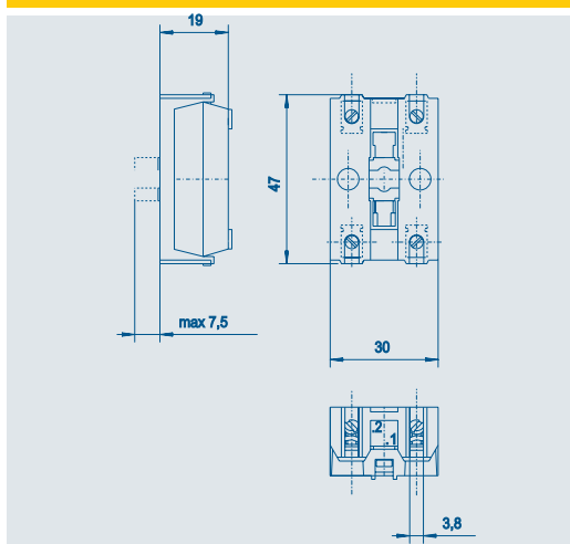
Wymiary gabarytowe członu łączeniowego EF30 Габаритные размеры коммутационного элемента EF30 Dimensions of contact block EF30
