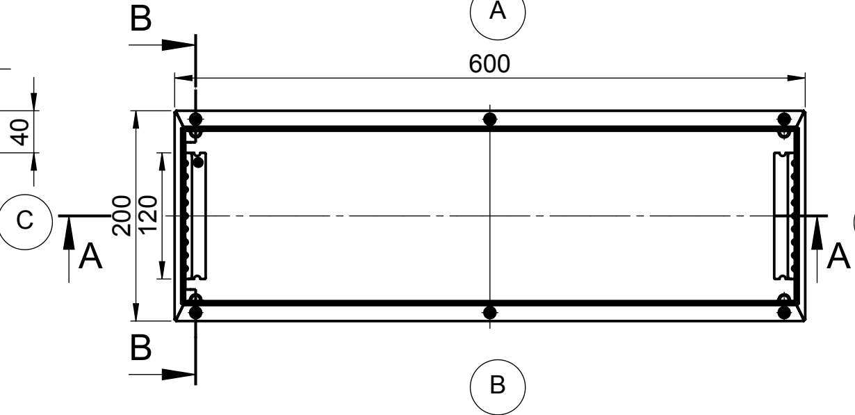
Unterteil / Base
