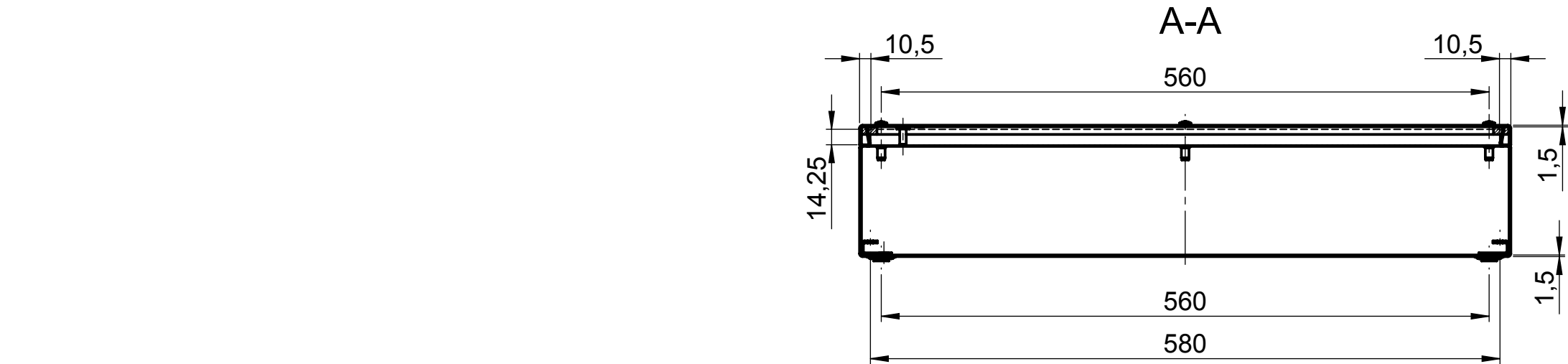
Unterteil / Base
