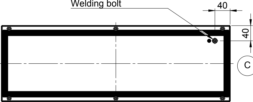
Deckel / Lid
