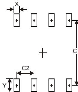
SO-8
