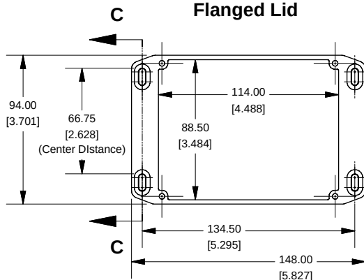
Flanged Lid
