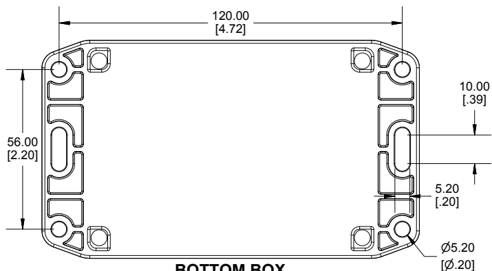
BOTTOM BOX
