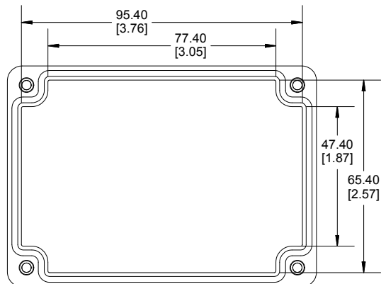
INSIDE LID
