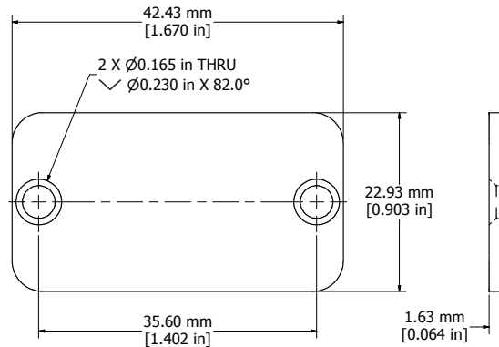
ENDPLATE
