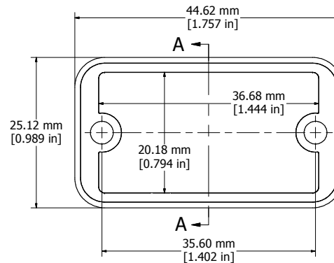
OPEN BEZEL
