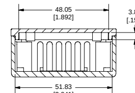
SECTION D-D
