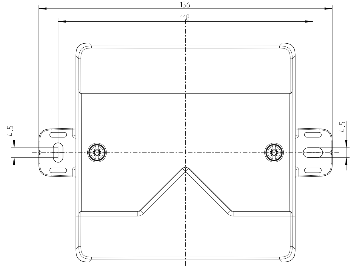
Mit Aussenbefestigungs-lasche/ with mounting lug
