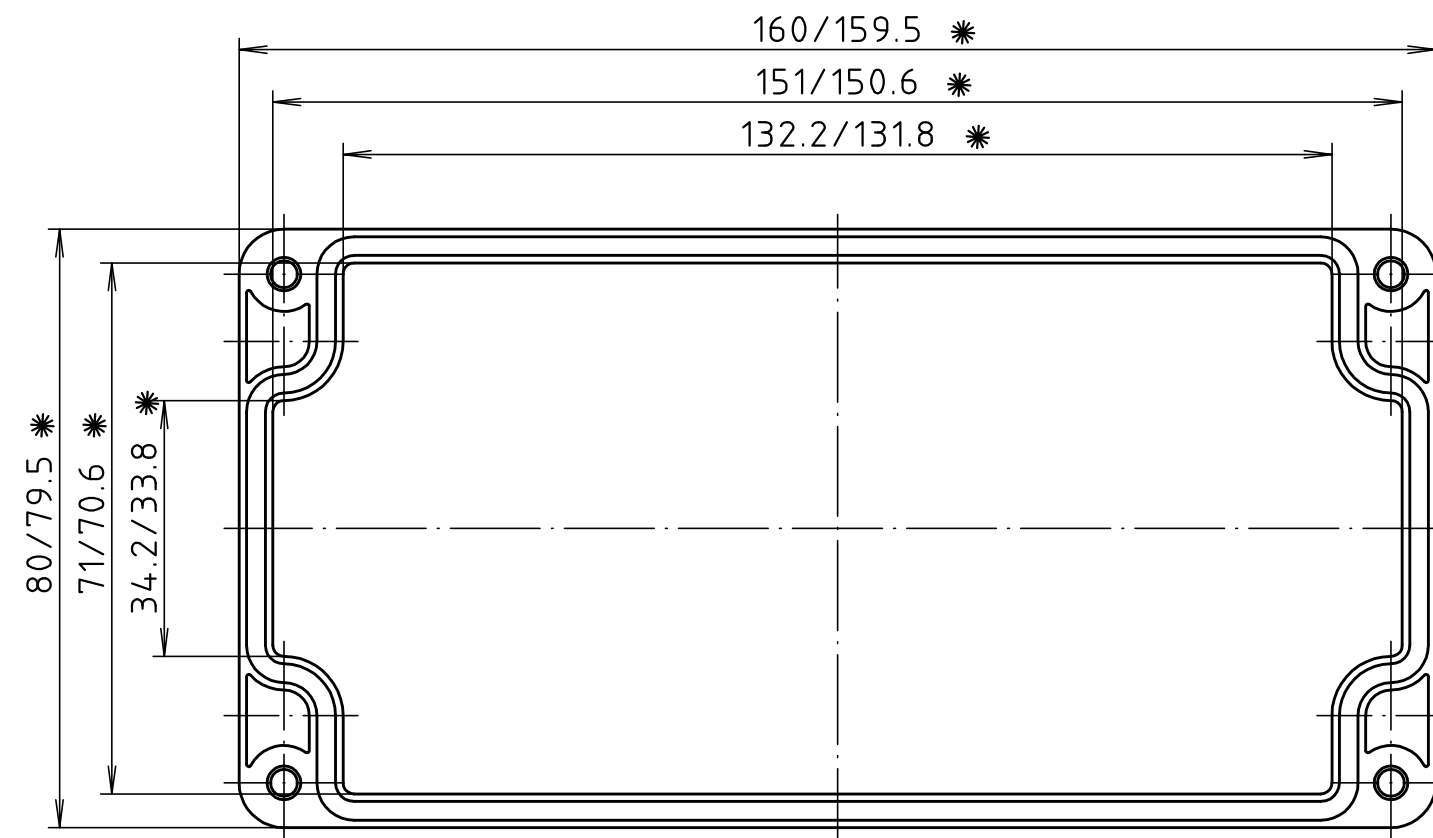
Deckel / lid
