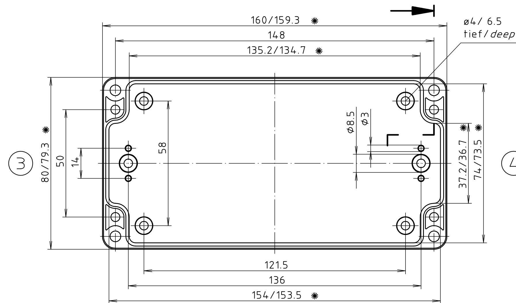
Unterteil / base
