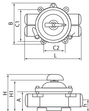
Исполнение 2, IP56 силюминовый корпус
