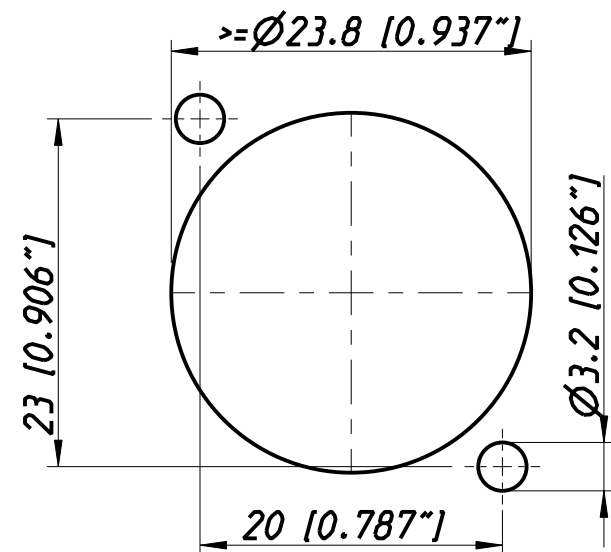
Frontplattenausschnitt (Frontseite) Panel cut out (front side)
