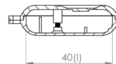
Sección/Section Q-Q
