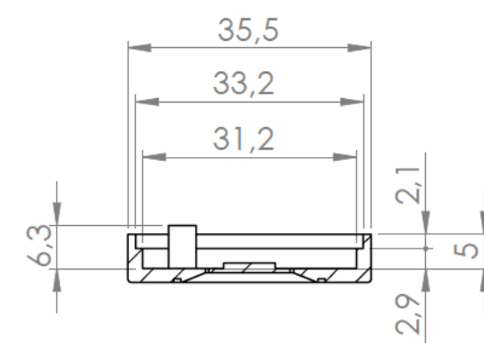
Sección/Section O-O
