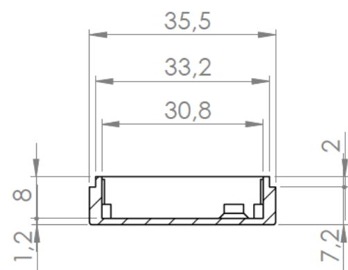
Sección/Section R-R
