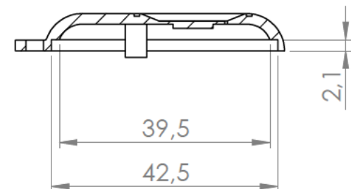
Sección/Section T-T
