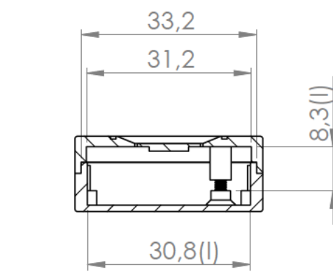
Sección/Section P-P
