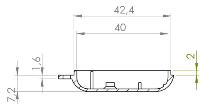
Sección/Section S-S
