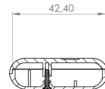
Sección /Section U-U
