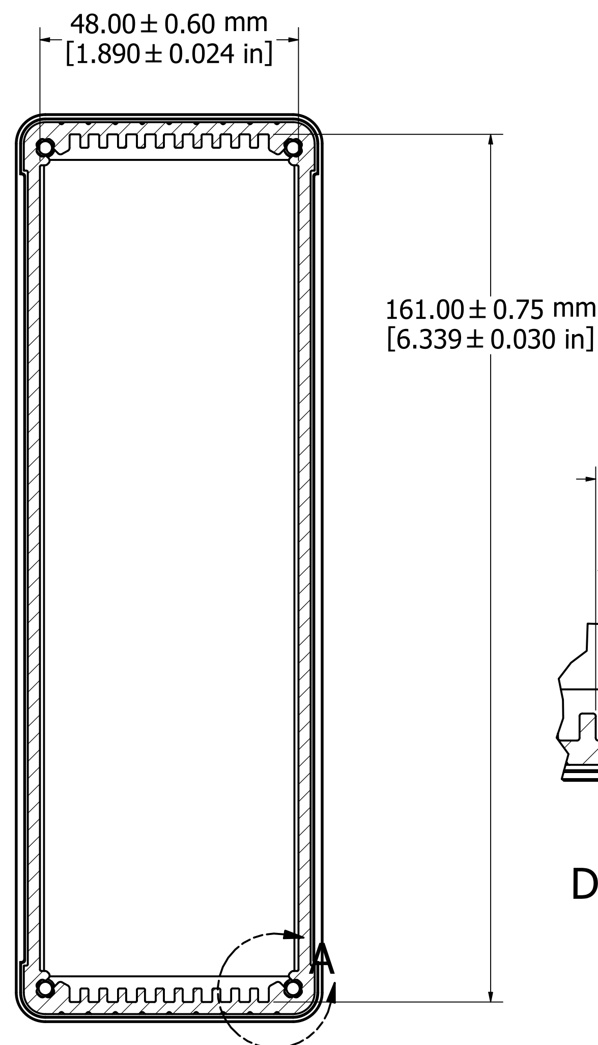
SECTION A-A
