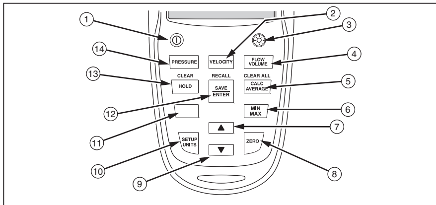
Abbildung 1. 922 Airflow Meter
