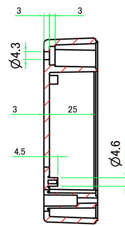
E-E ( 1 : 2 )
