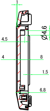
C-C ( 1 : 2 )
