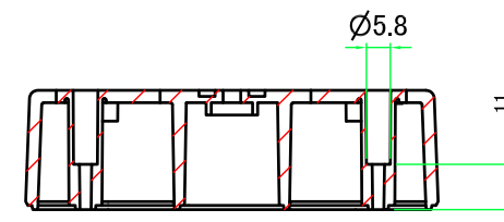
F-F ( 1 : 2 )
