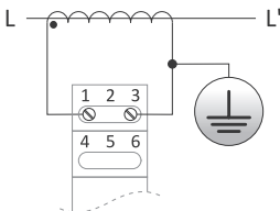
Pośredni pomiar natężenia prądu z wykorzystaniem przekładników prądowych
