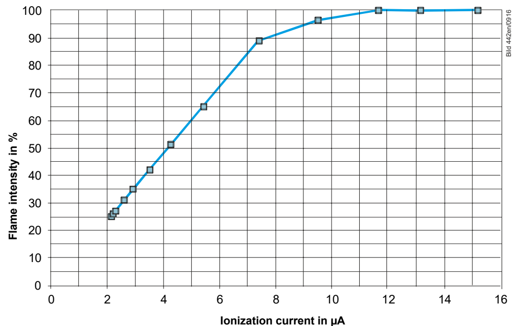
Ionization input
