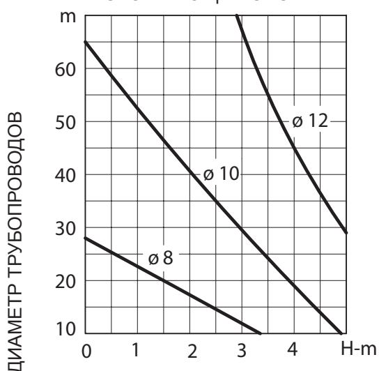
ВСАСЫВАЮЩАЯ СИСТЕМА
