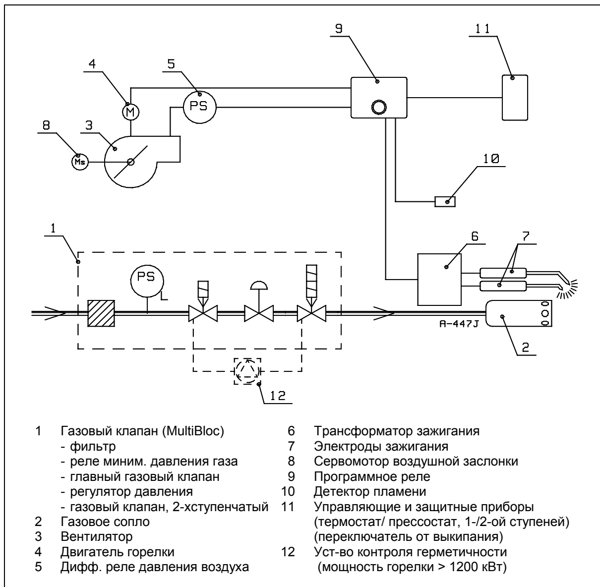
Схема № А-447J
