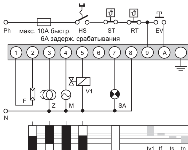
Схема соединений и диаграмма протекания программного цикла для DKO 972 (кроме Mod.25)
