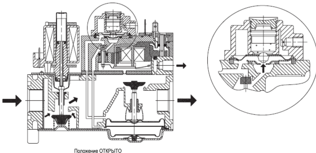
Положение ОТКРЫТО
