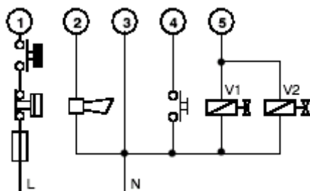
Рис. 12. Схема соединений S4560B, Q* с подключением реле пламени с обесточенными контактами
