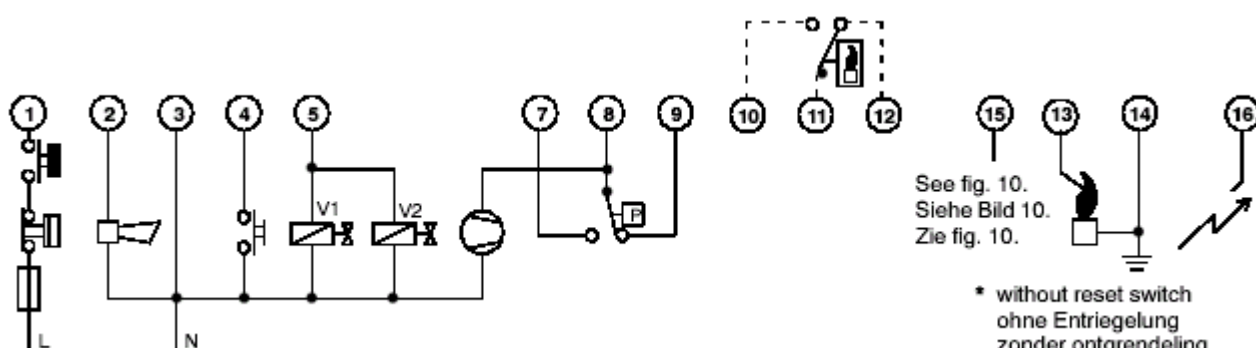
Рис. 17. Схема соединений S4560D, T* с подключением реле пламени с обесточенными контактами
