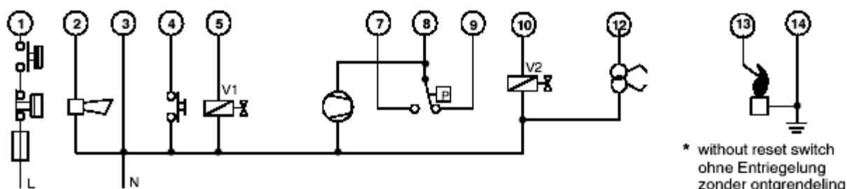
Рис. 18. Схема соединений S4560D, T*
