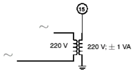
Рис. 10. Применение S4560A ... T при плавающем напряжении сети
