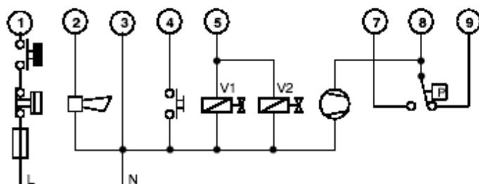
Рис. 16. Схема соединений S4560C, R*
