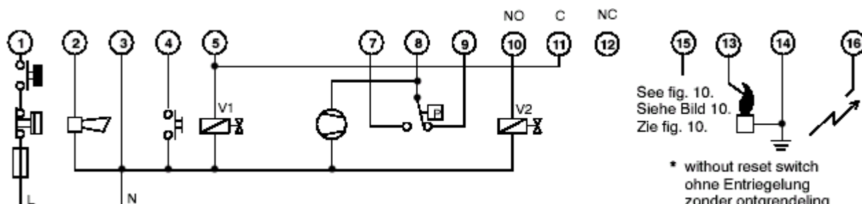
Рис. 17. Схема соединений S4560D, T* с подключением реле пламени с обесточенными контактами
