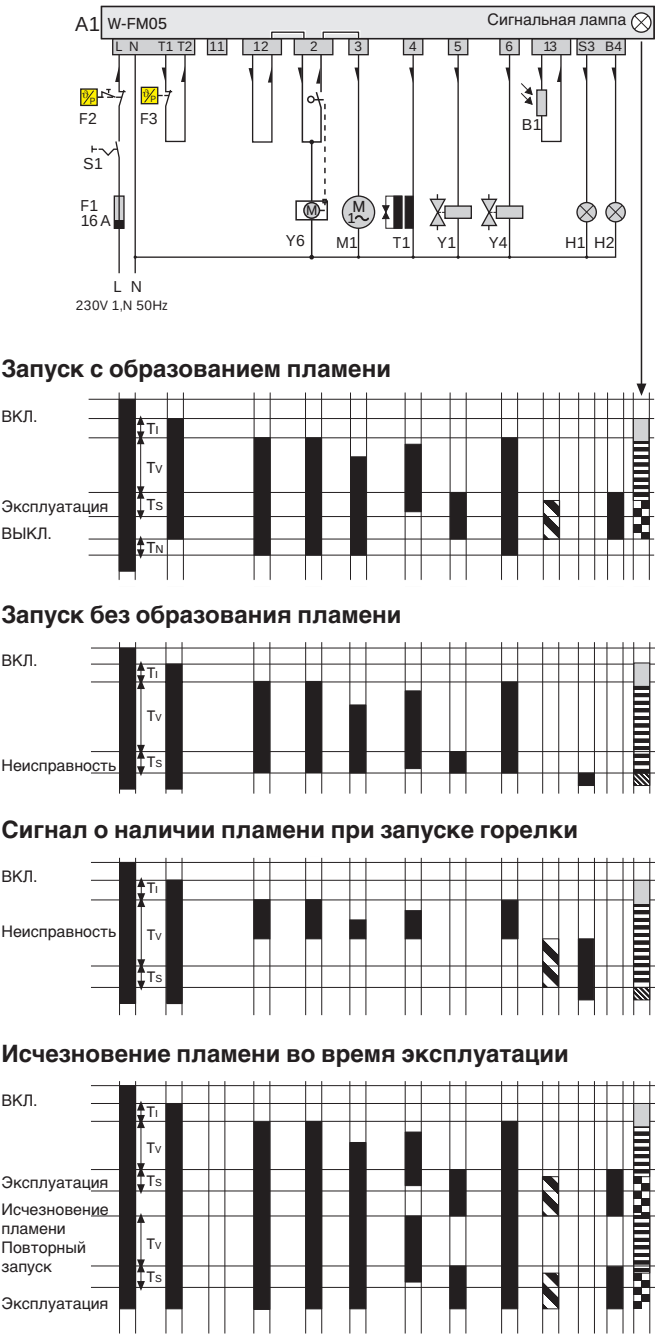
Диаграмма последовательности действий
