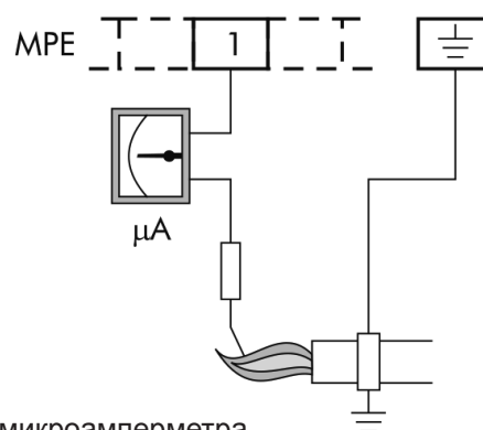
Присоединение микроамперметра
