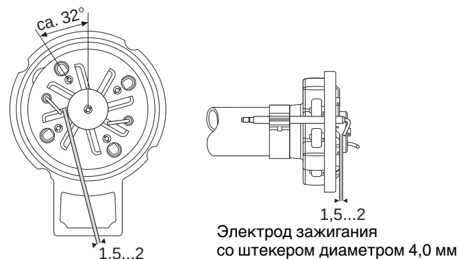
Установочные размеры для электрода зажигания
