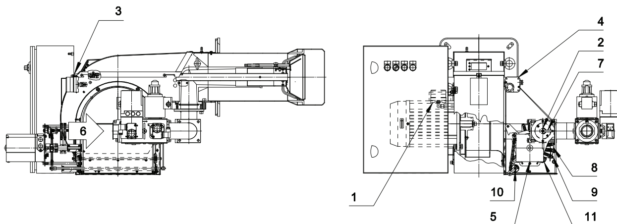
Fig. 12 РЕГУЛИРОВКА ГОРЕЛКИ
