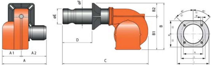
Габариты
