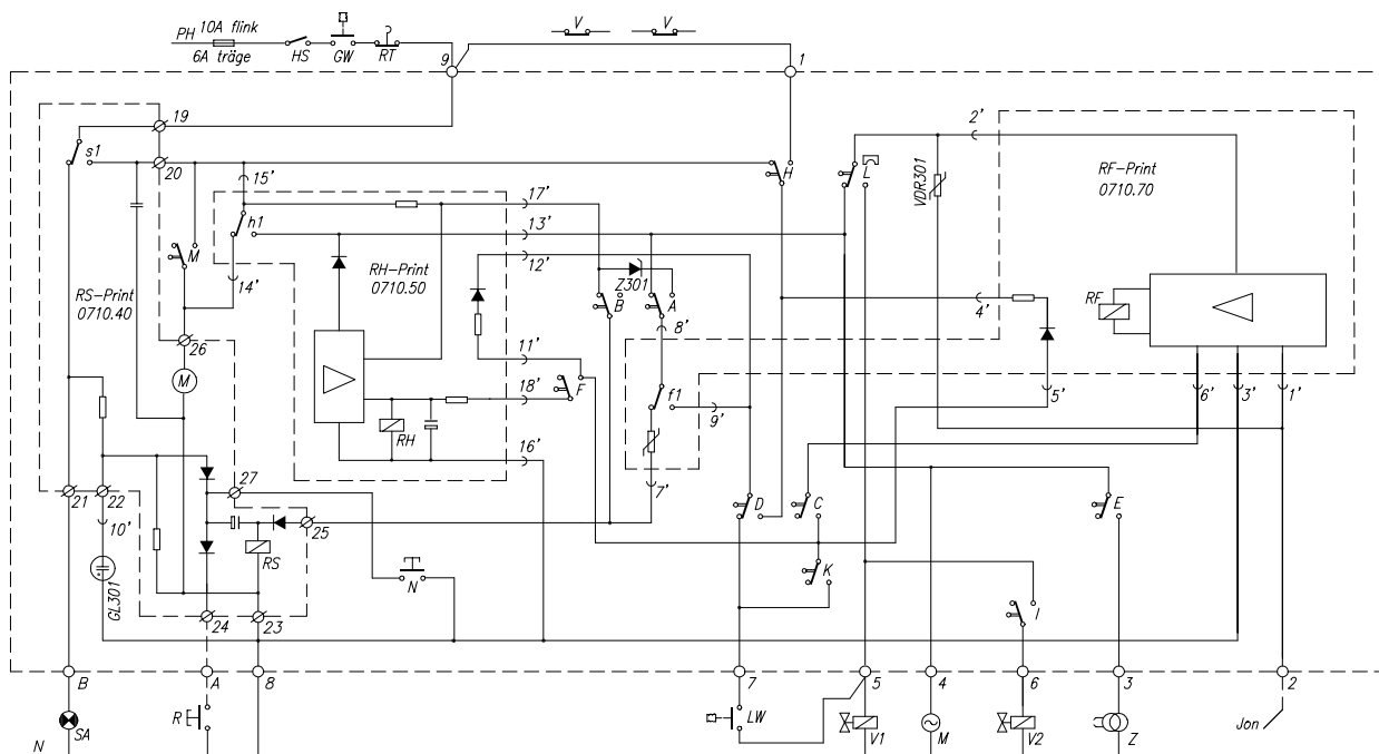
Электросхема MMI 810.1
