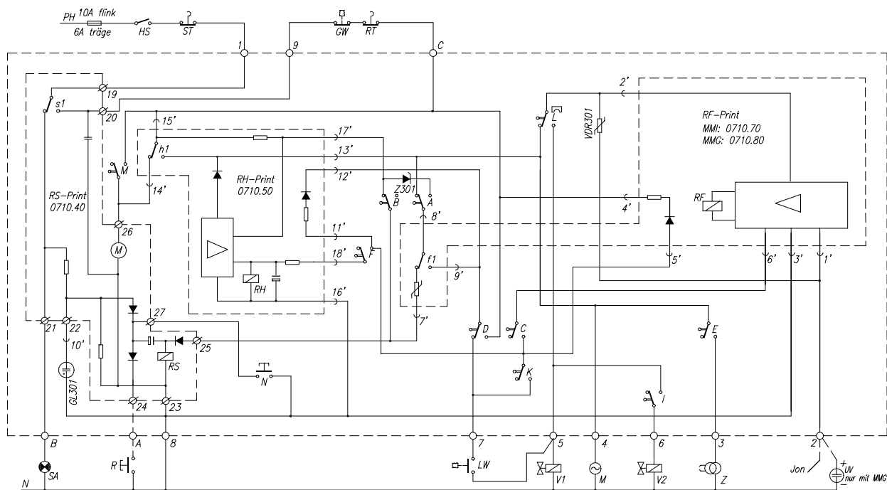
Электросхема MMI 811.1
