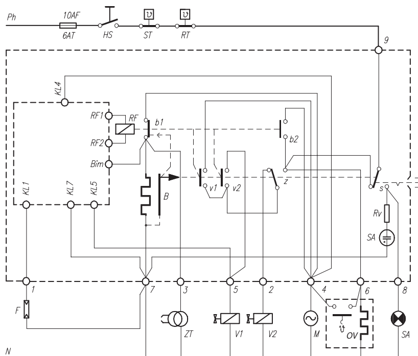
Электросхема TFI 976
