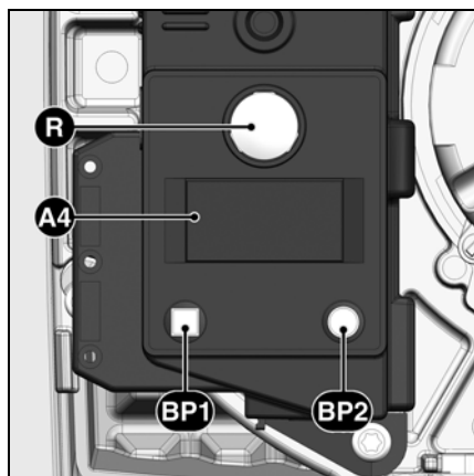
A4 Дисплей BP1 Кнопка 1 Опрос: код неисправности BP2 Кнопка 2 Опрос: значение
