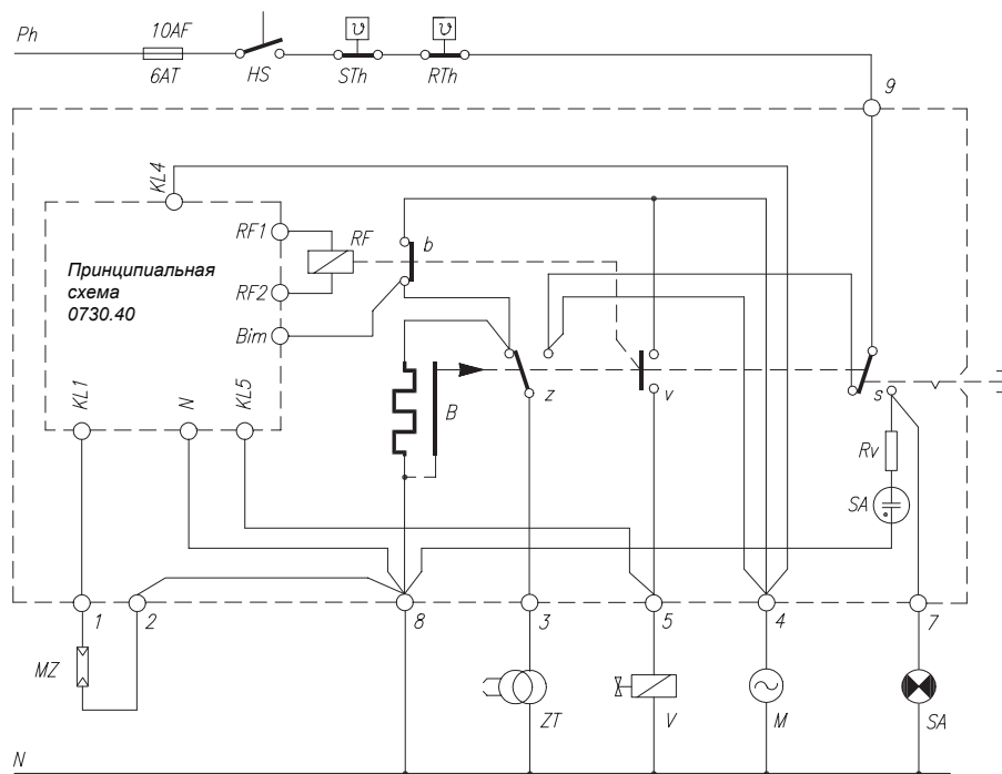
Электросхема TFI 830.3
