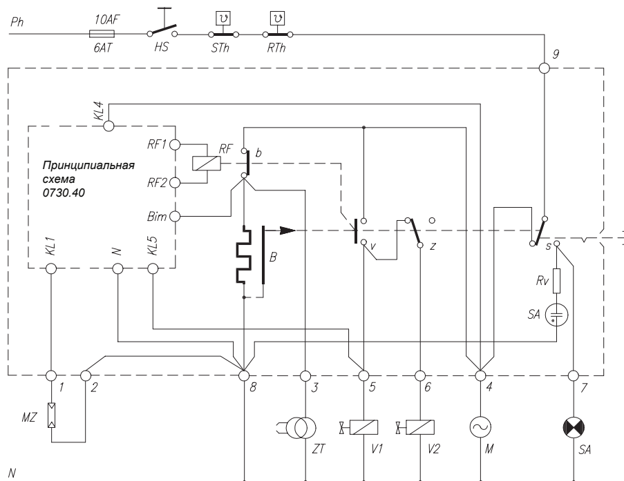
Электросхема TFI 832.3
