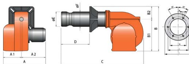
Габариты
