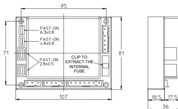
Рис. 1 – Габаритные размеры
