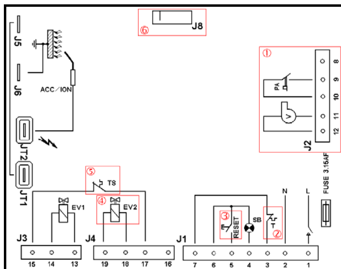
Тип DTMN32 в исполнении с моноэлектродом
