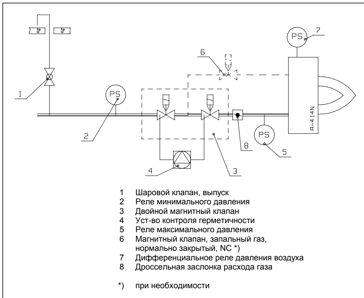
Схема № А-414N
