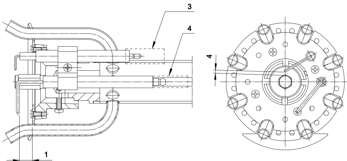
Fig. 14 УСТАНОВКА ЭЛЕКТРОДОВ
