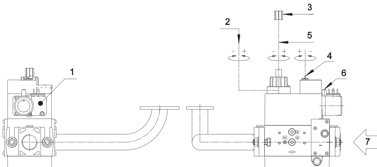
Fig. 12 РЕГУЛИРОВКА ГАЗОВОЙ АРМАТУРЫ МОД.: DUNGS
