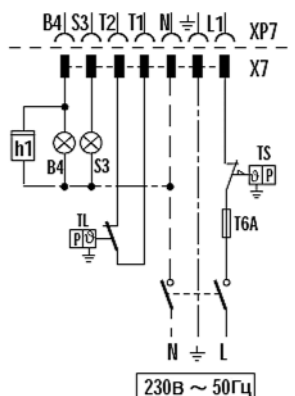
Электрическая схема горелки
