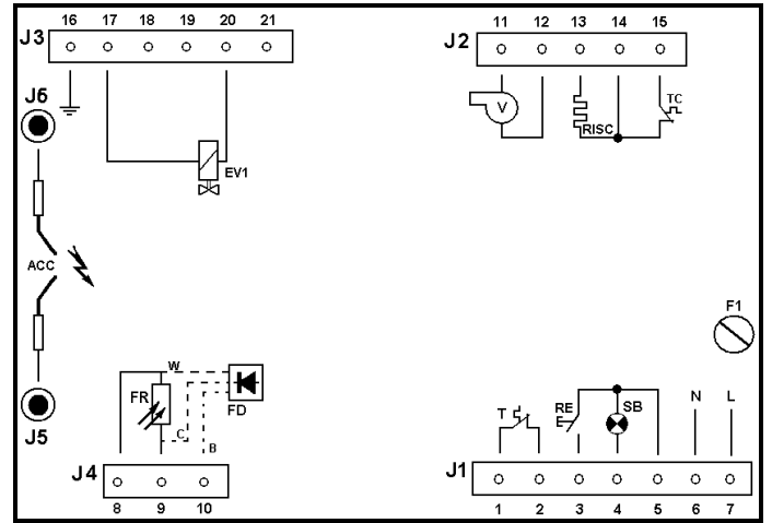
Type TGRD71
