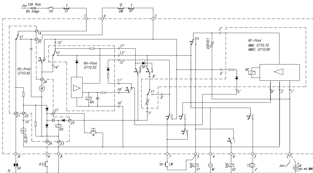
Электросхема MMI 811.1
