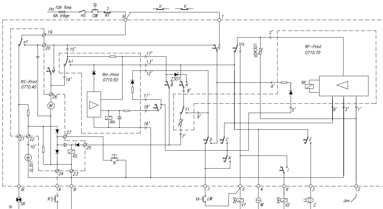
Электросхема MMI 810.1
