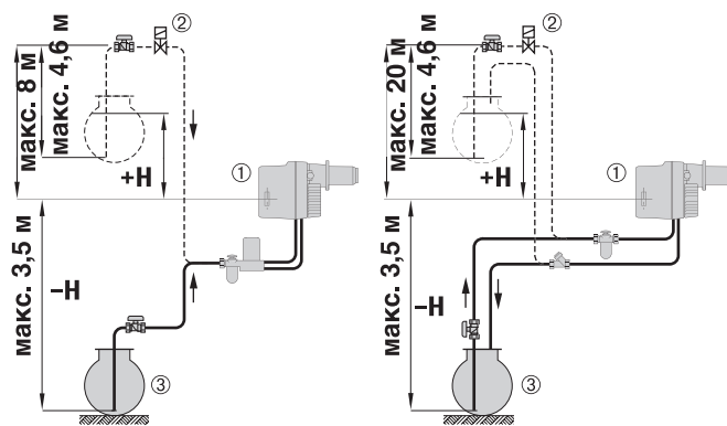
Одноструйная система
