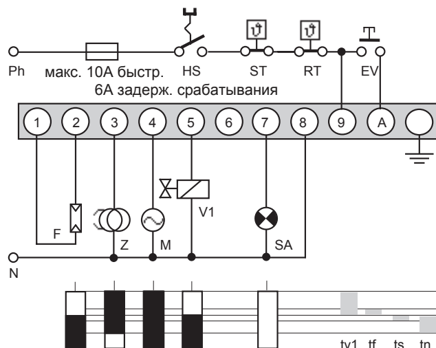
Схема соединений и диаграмма протекания программного цикла для DKO 970
