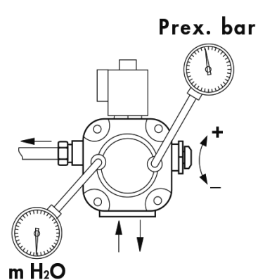
DELTA- VM 1
